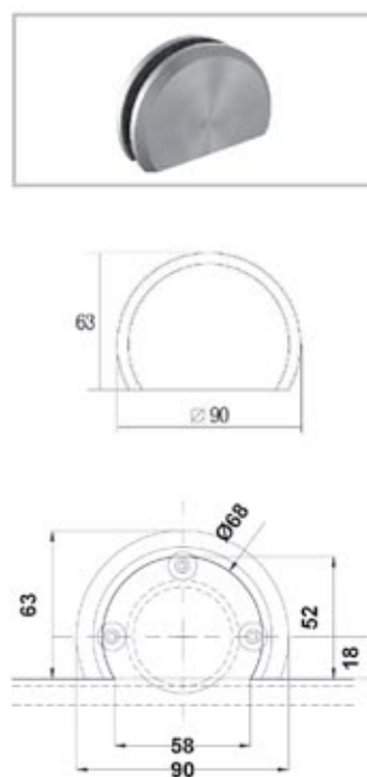
BRK 3330 Carretilla sencilla para riel inferior. Carga máxima de 35 Kg
