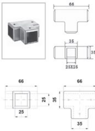
BRK 3809 Conector t cuadrado para tres barras.
