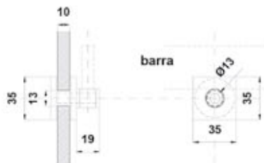
BRK 3850-1I. Conector barra cuadrada a muro.
