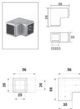
BRK 3808 Conector cuadrado para doble barra a 90°.
