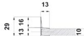
BRK 3850-1L. Botaguas con aleta a 90°.
