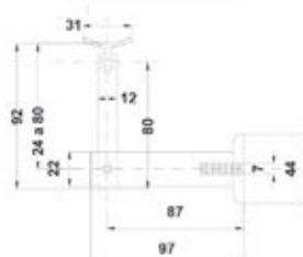
BRK 3042-4 Conector de poste para barandal a pasamanos plano.
