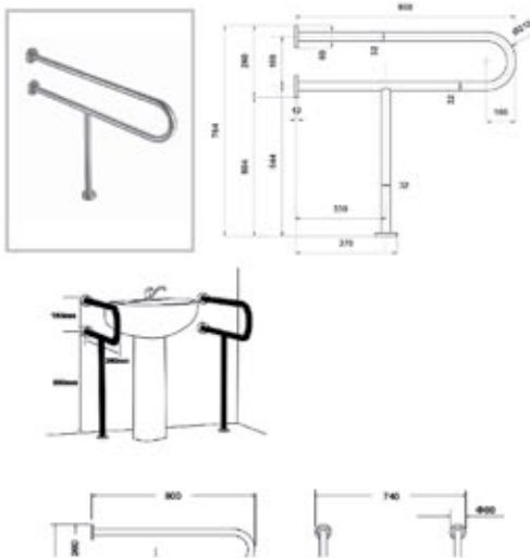
BRK 3822 Barra estabilizadora *t+u* 90° para lavabo 32 mm.
