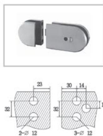
■ BRK 3805 Seguro cristal - cristal con resaque con indicador de posición.
