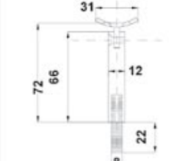
BRK 3042-8 Conector de poste para barandal a pasamanos redondo con rosca incluida.
