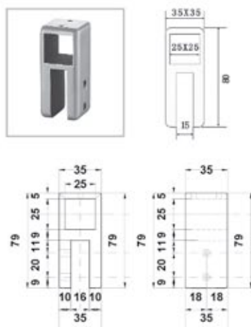
■ BRK 3807 Conector cuadrado cristal a barra.
