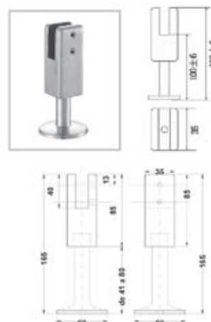
■ BRK 3806 Soporte cuadrado para panel de cristal con sujeción a piso 8-12mm.
