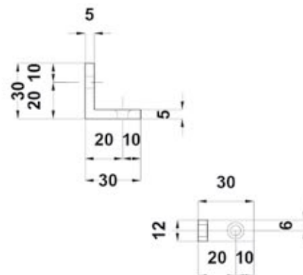
BRK 3930B-07. Escuadra de armado.
