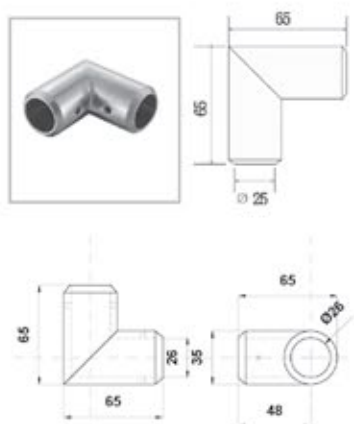
BRK 3803 Conector redondo para doble barra a 90°.
