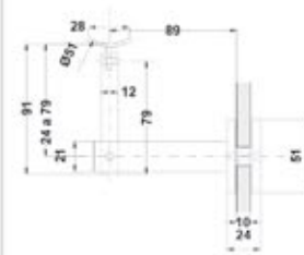
BRK 3042-2 Conector articulado de poste para barandal a pasamanos redondo.
