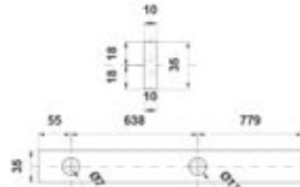
BRK 3850-1K. Barra de acero 304 acabado en satin o en cromo.
