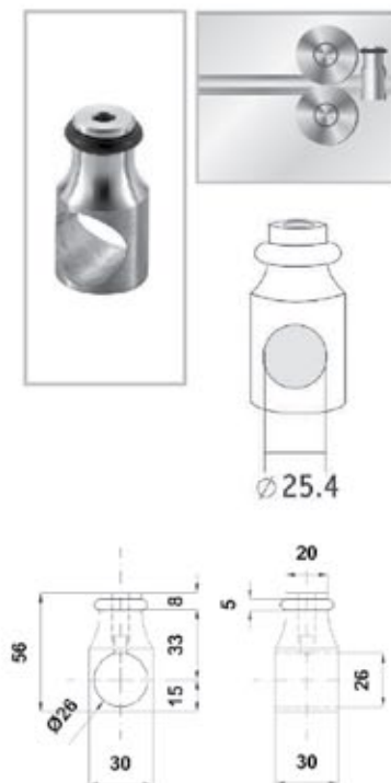
BRK 3324 Tope para doble carretilla BR3311C. Fijación a tubo.
