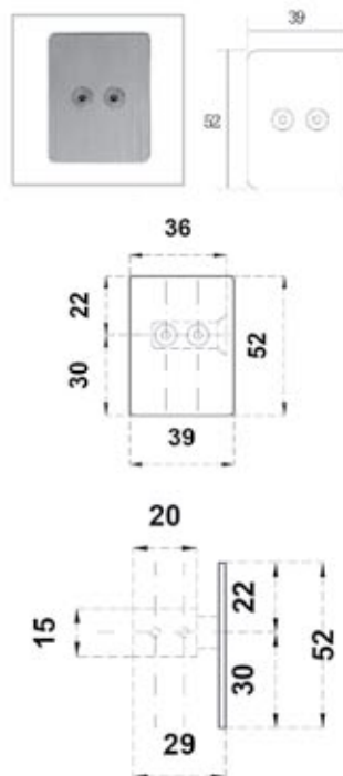
BRK 3335 Tapa final de riel superior con fijación a riel superior.
