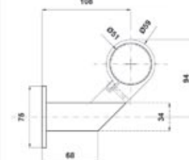
BRK 3042-3 Conector articulado de poste para barandal a pasamanos redondo con rosca incluida.
