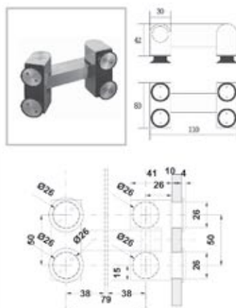
BRK 3718 Bisagra cristal a 180° doble acción para 25kg.
