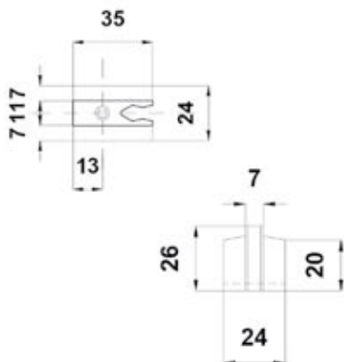
BRK 3930B-04. Tope con instalación en riel.
