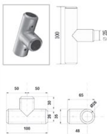
BRK 3804 Conector t redondo para tres barras.
