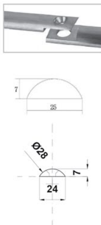
BRK 3331 Riel inferior para carretilla sencilla media luna de 2 mts.
