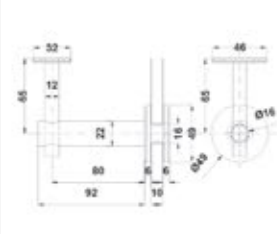
BRK 3042-6 Conector articulado de poste para barandal a pasamanos plano.
