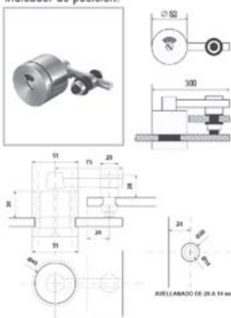
BRK 3812 Seguro cristal - cristal con traslape con perforación a cristal con indicador de posición.
