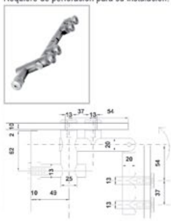
BRK 3813 Bisagra para puerta abatible y fijo con fijación cristal-cristal. Requiere de perforación para su instalación.
