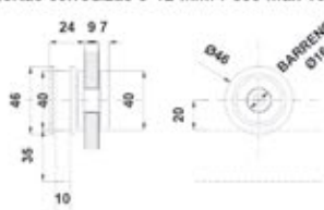
BRK 3850-1J. Carretilla sencilla con sujeción a cristal para barra cuadrada de sistemas de puertas corredizas 8-12 mm. Peso máx 100 kg.
