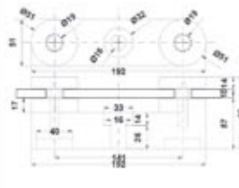
BRK 3762-1A Adaptador circular para barandal plano.
