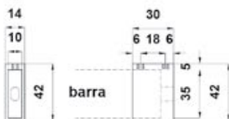
BRK 3850-1I. Conector barra cuadrada a muro.
