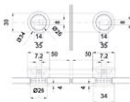
BRK 3699 Llave ajustable para conectores con nariz de puerco.
