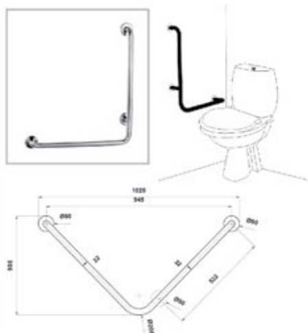
BRK 3821 Barra estabilizadora 1" 90° para baño 32 mm.
