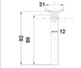
BRK 3042-7 Conector de poste para barandal a pasamanos redondo.
