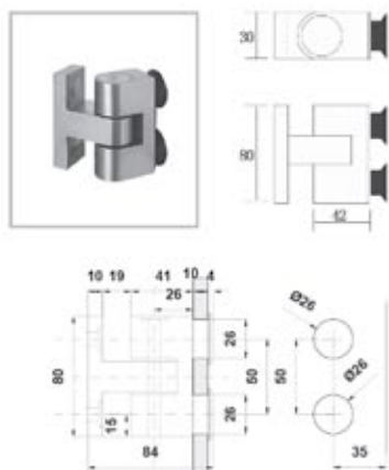
BRK 3712 Bisagra muro vidrio peso máximo 25kg.
