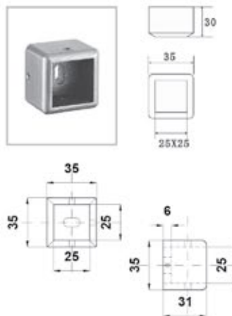
■ BRK 3810 Conector para barra cuadrada con fijación a muro.
