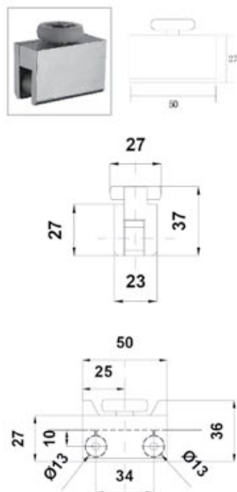
BRK 3333 Carretilla para riel superior con clip a cristal.
