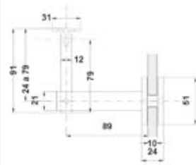
BRK 3042-1 Conector base redonda de cristal a pasamanos plano.
