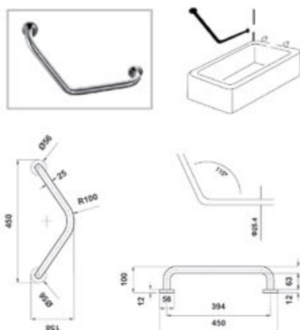
BRK 3820 Barra estabilizadora 1" 135° para tina/regadera 25.4 mm.
