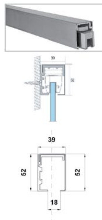
BRK 3332 Riel superior de sujeción a muro de 2 mts.
