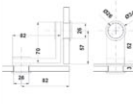
BRK 3761B Conector piso o techo 90°.
