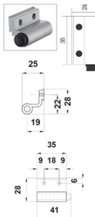
BRK 3334 Tope para puerta corrediza con fijación a riel superior.
