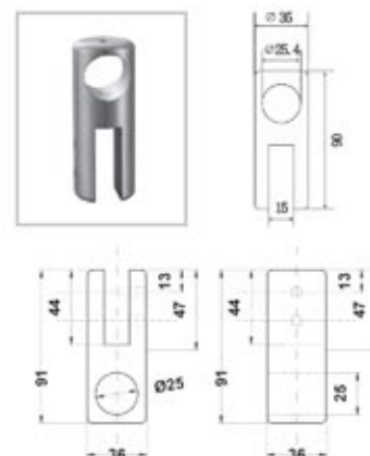
BRK 3802 Conector redondo cristal a barra.
