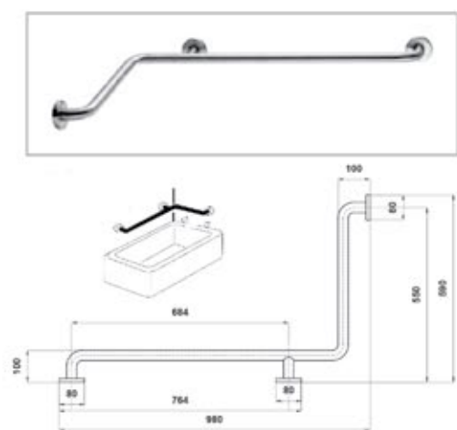
BRK 3819 Barra estabilizadora "T" 90° para tina/regadera 32mm.
