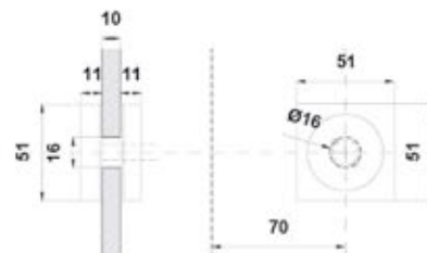
BRK 3850-1L. Botaguas con aleta a 90°.
